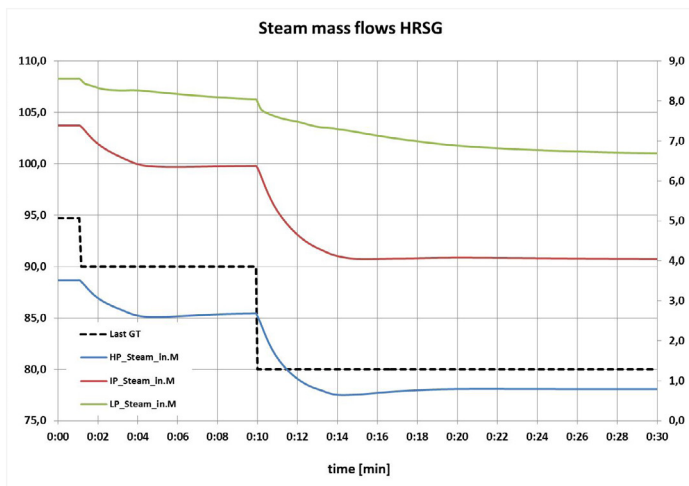
Zeitentwicklung der Dampfströme vom Abhitzekeessel einer GUD-Anlage
