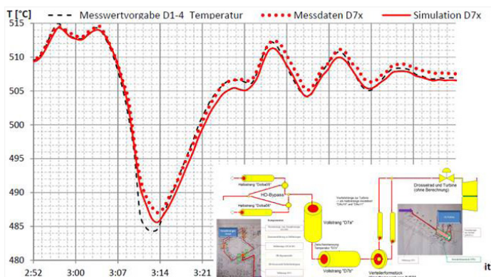
Dynamische Simulation einer Frischdampfleitung
